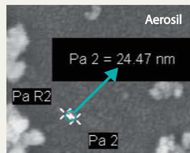
<SEM images of Fillers: B.G & Aerosil>
