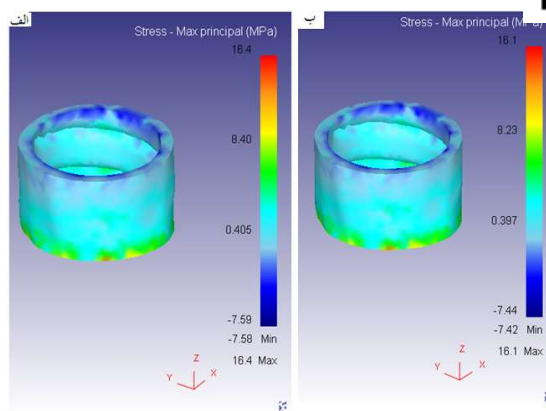
شکل ۵- توزیع تنش‌های ماکزیم اصلی در دو مدل استخوان کورتیکال تازه تشکیل شده پس از بارگذاری در مجاورت ایمپلنت، الف) تیتانیوم خالص و ب) زیرکونیوم -۲/۵٪ نایوبیوم
