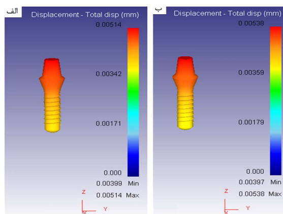
شکل ۶- شماتیکی از توزیع جابه جایی در ایمپلنت الف) تیتانیوم خالص، ب) زیرکونیوم -۲/۵٪ نایوبیوم
