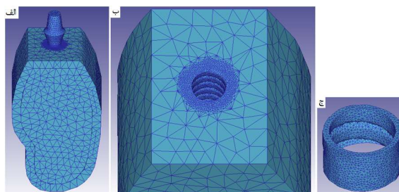
شکل ۴- الف) مدل ایمپلنت ITI قرار داده شده در استخوان فک ب) جدا کردن هندسه ایمپلنت از مدل کنسولوس استخوان فک با دستورالعمل Boolean operation، ج) جدا کردن هندسه ایمپلنت از مدل سه بعدی حفره ایجاد شده روی مدل استخوان کورتیکال تازه تشکیل شده با دستورالعمل Boolean operation
